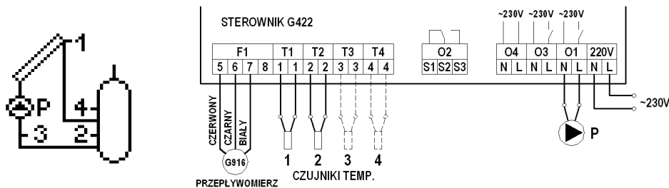
Rys. 3. Schemat ideowy oraz elektryczny instalacji nr 1.
