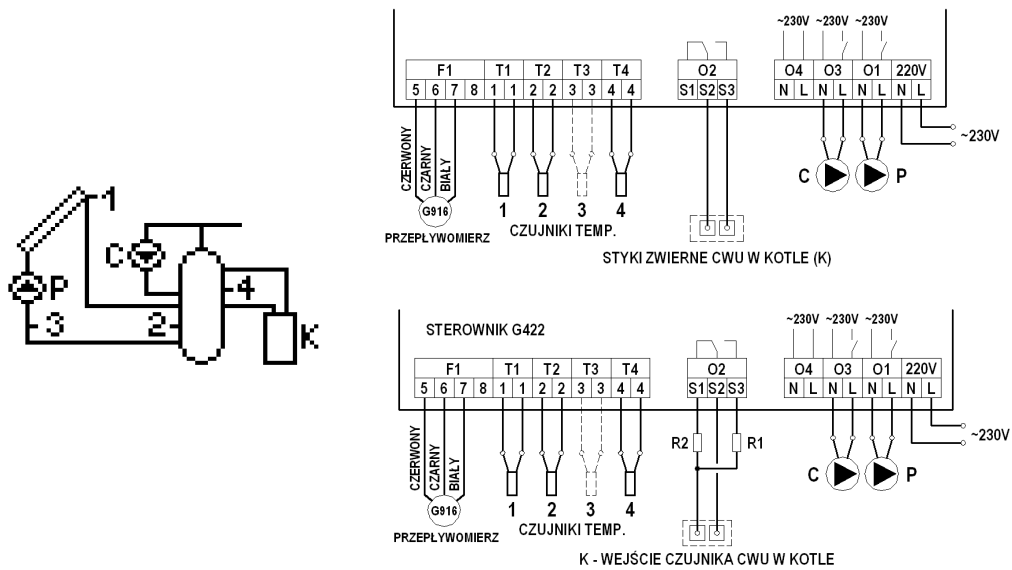
Rys. 5. Schemat ideowy oraz elektryczny instalacji nr 3.
