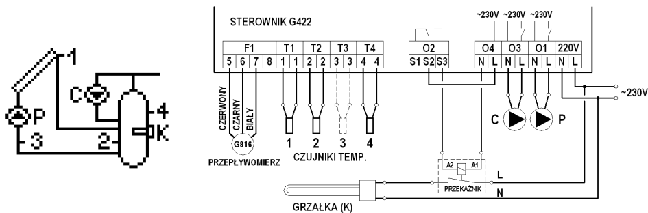
Rys. 6. Schemat ideowy oraz elektryczny instalacji nr 4.
