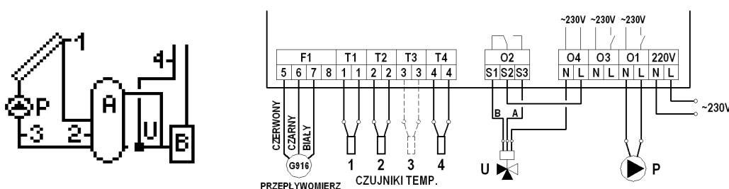
Rys. 15. Schemat ideowy oraz elektryczny instalacji układu nr 7.
