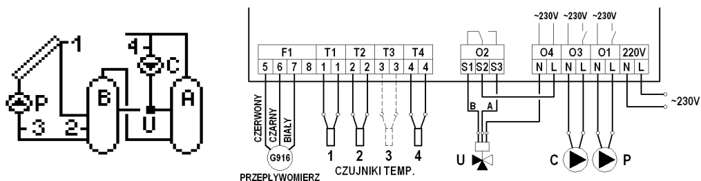
Rys. 10. Schemat ideowy oraz elektryczny instalacji układu nr 8.
