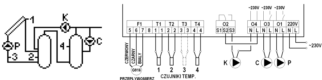
Rys. 9. Schemat ideowy oraz elektryczny instalacji nr 7.
