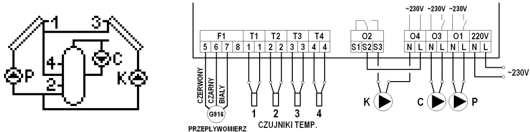
Rys. 17. Schemat ideowy oraz elektryczny instalacji układu nr 15.
