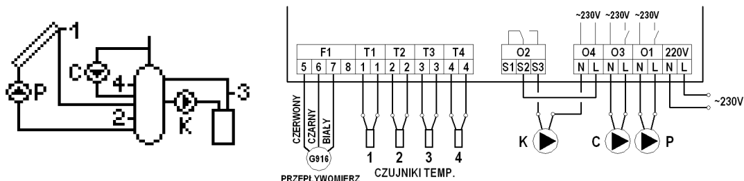
Rys. 8. Schemat ideowy oraz elektryczny instalacji nr 6.
