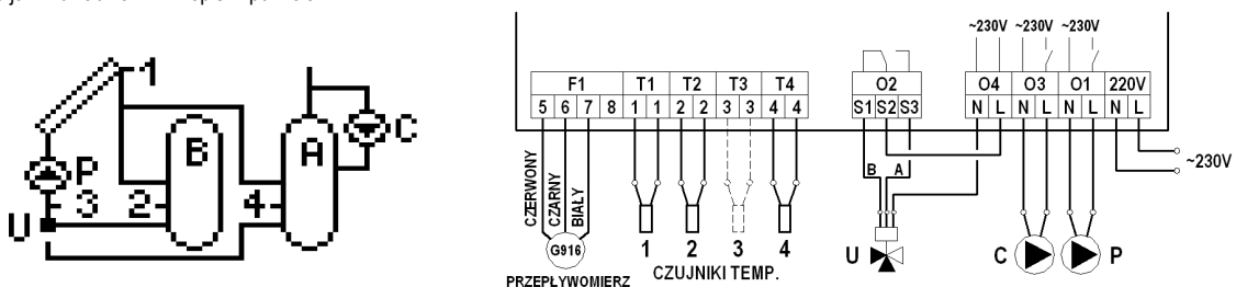
Rys. 13. Schemat ideowy oraz elektryczny instalacji układu nr 11.
