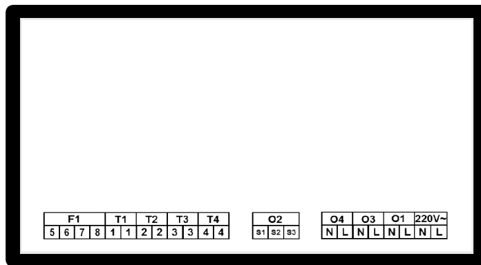
Rys. 1. Oznaczenie wejść i wyjść sterownika.
