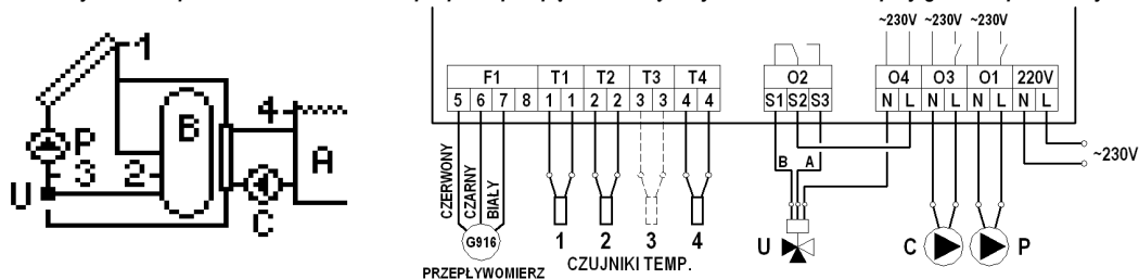
Rys. 11. Schemat ideowy oraz elektryczny instalacji nr 9.
