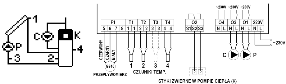
Rys. 7. Schemat ideowy oraz elektryczny instalacji nr 5.
