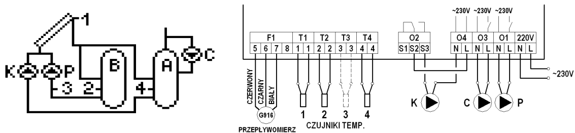
Rys. 14. Schemat ideowy oraz elektryczny instalacji układu nr 12.
