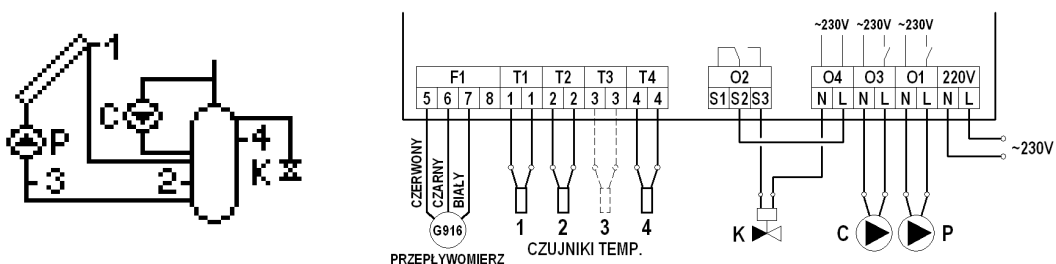
Rys. 19. Schemat ideowy oraz elektryczny instalacji układu nr 17.
