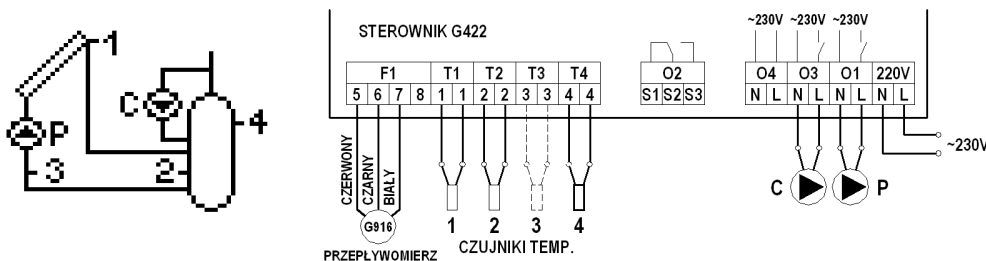
Rys. 4. Schemat ideowy oraz elektryczny instalacji nr 2.
