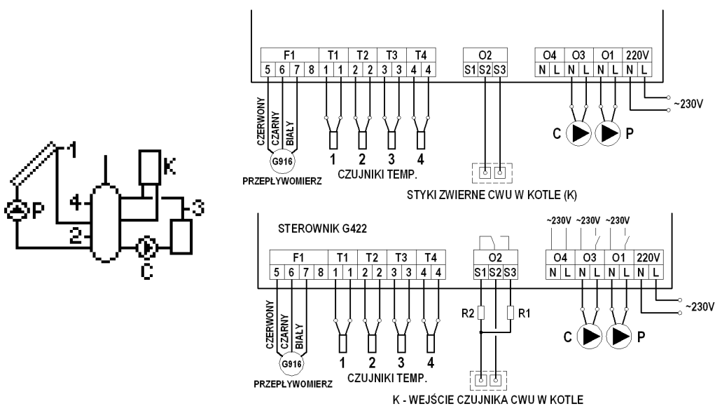
Rys. 16. Schemat ideowy oraz elektryczny instalacji układu nr 14.
