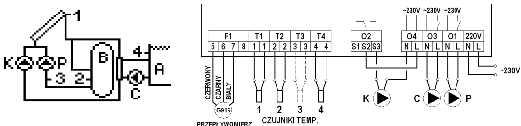
Rys. 12. Schemat ideowy oraz elektryczny instalacji nr 10.
