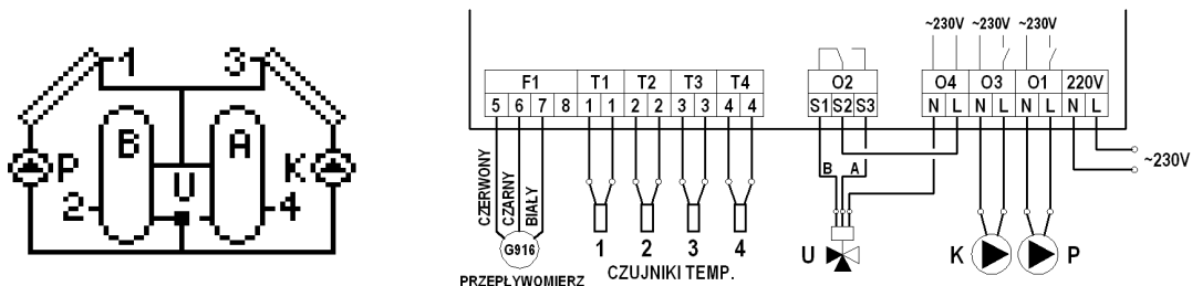
Rys. 18. Schemat ideowy oraz elektryczny instalacji układu nr 16.
