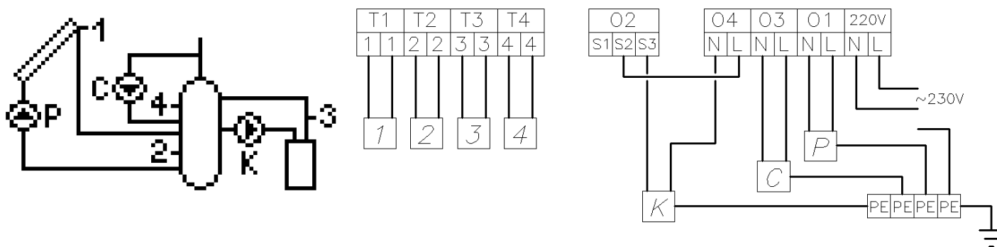
Rys. 15. Schemat ideowy oraz elektryczny instalacji nr 6.
