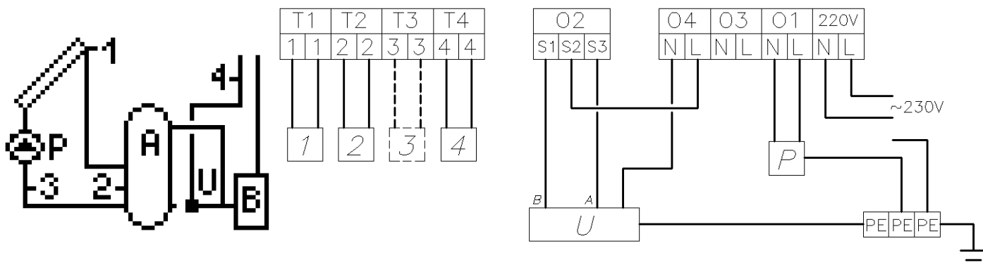
Rys. 22. Schemat ideowy oraz elektryczny instalacji układu nr 7.
