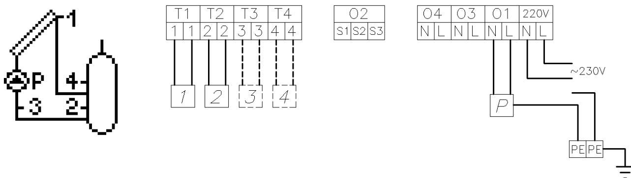
Rys. 10. Schemat ideowy oraz elektryczny instalacji nr 1.
