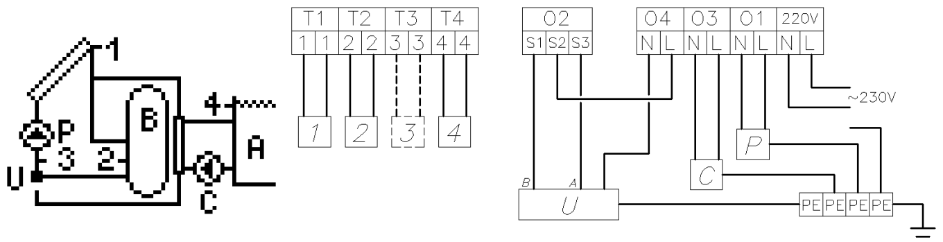
Rys. 18. Schemat ideowy oraz elektryczny instalacji nr 9.
