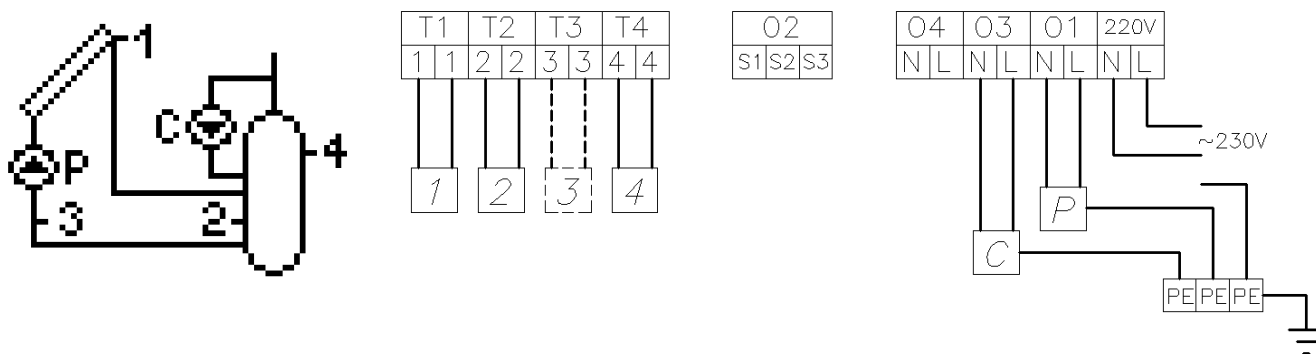
Rys. 11. Schemat ideowy oraz elektryczny instalacji nr 2.
