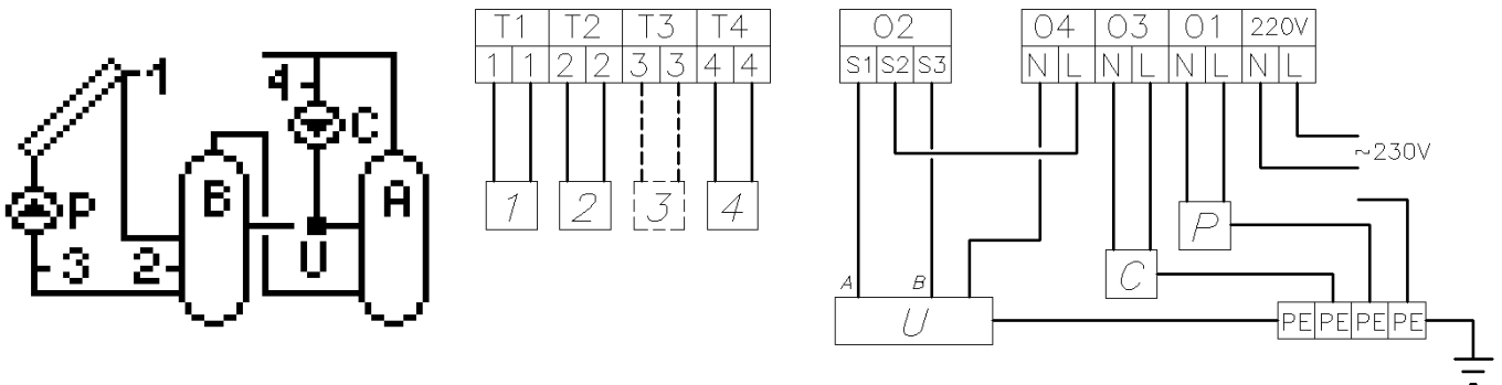
Rys. 17. Schemat ideowy oraz elektryczny instalacji układu nr 8.
