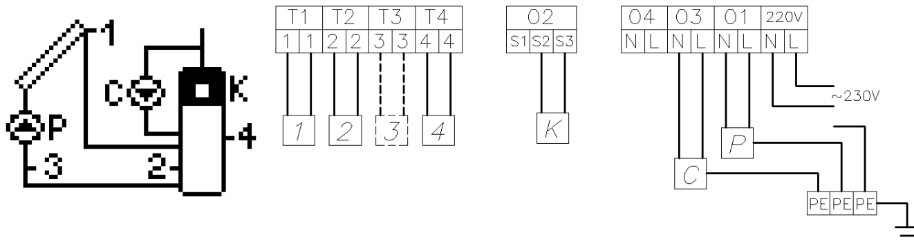
Rys. 14. Schemat ideowy oraz elektryczny instalacji nr 5.
