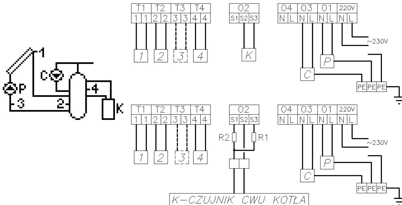
Rys. 12. Schemat ideowy oraz elektryczny instalacji nr 3.
