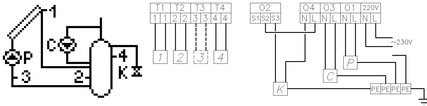
Rys. 26. Schemat ideowy oraz elektryczny instalacji układu nr 17.
