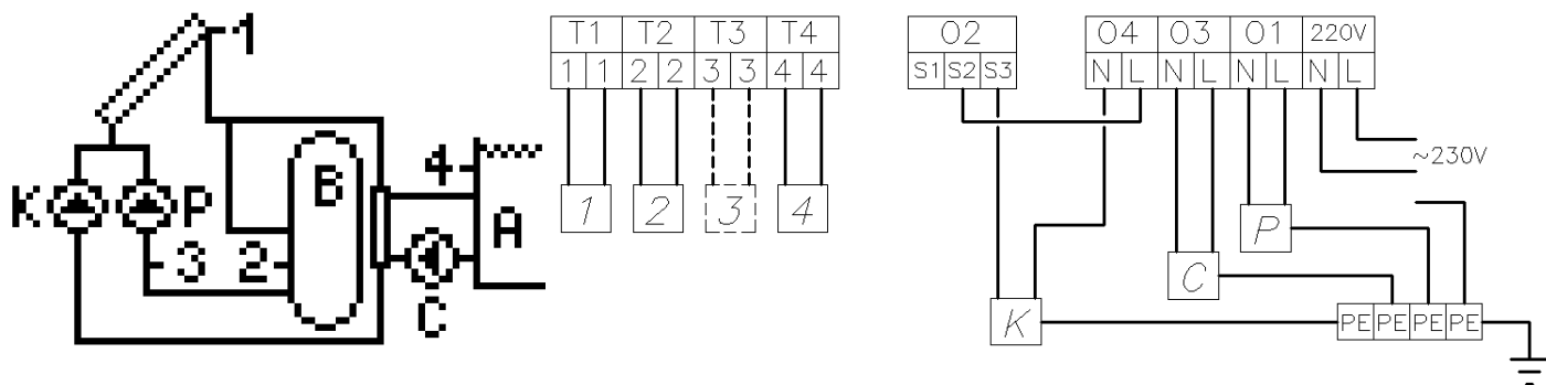
Rys. 19. Schemat ideowy oraz elektryczny instalacji nr 10.
