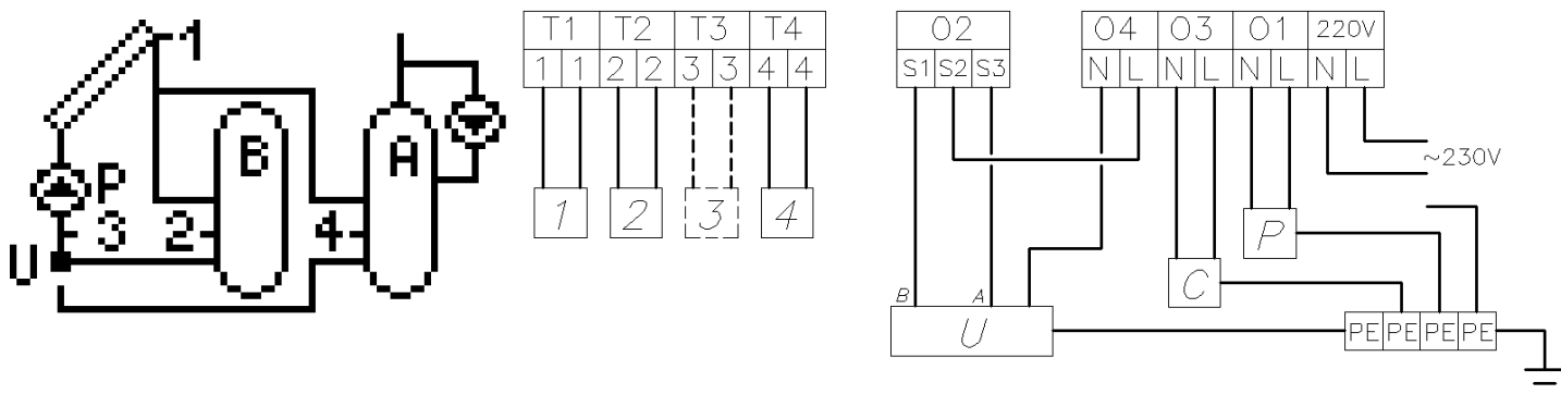
Rys. 20. Schemat ideowy oraz elektryczny instalacji układu nr 11.
