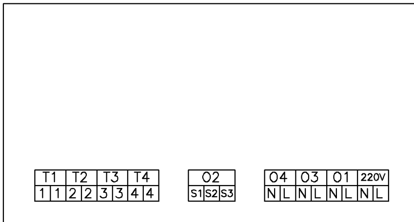
Rys. 1. Oznaczenie wejść i wyjść sterownika.
