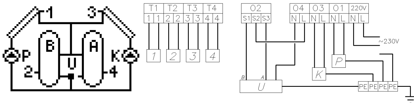
Rys. 25. Schemat ideowy oraz elektryczny instalacji układu nr 16.
