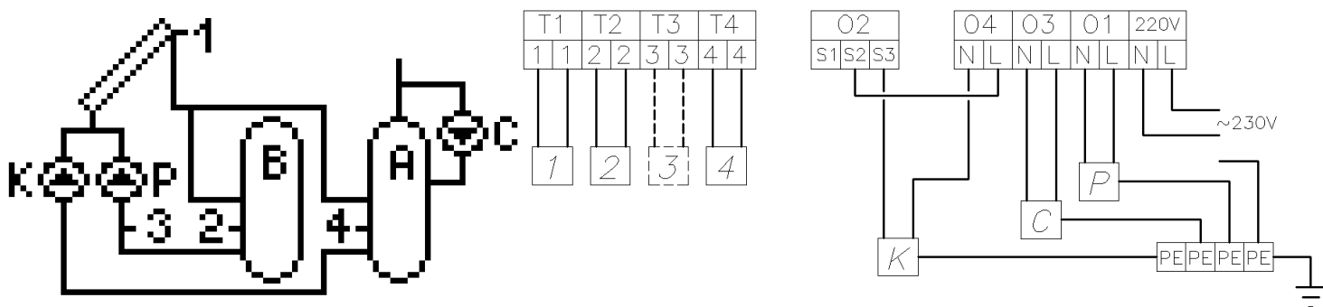
Rys. 21. Schemat ideowy oraz elektryczny instalacji układu nr 12.
