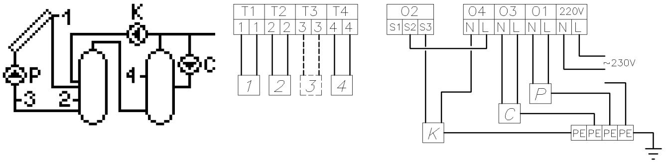
Rys. 16. Schemat ideowy oraz elektryczny instalacji nr 7.
