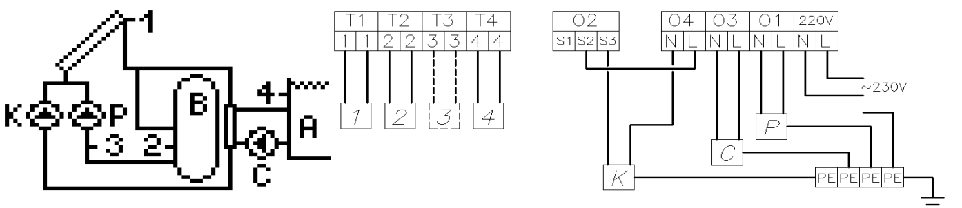
Rys. 19. Schemat ideowy oraz elektryczny instalacji nr 10.
