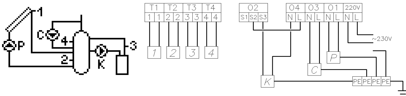
Rys. 15. Schemat ideowy oraz elektryczny instalacji nr 6.
