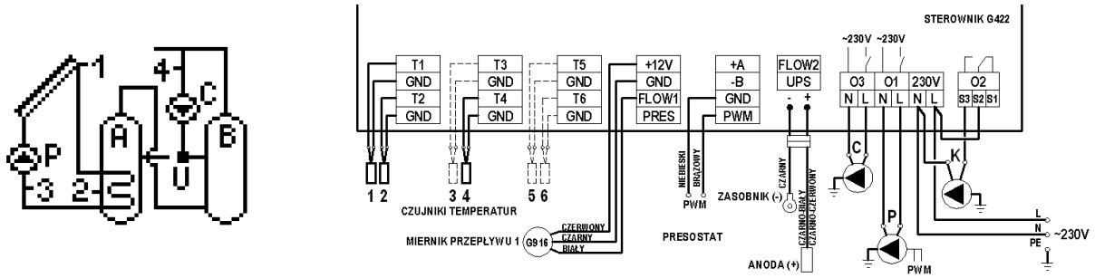
Schemat 8. Schemat ideowy oraz elektryczny instalacji układu nr 8.
