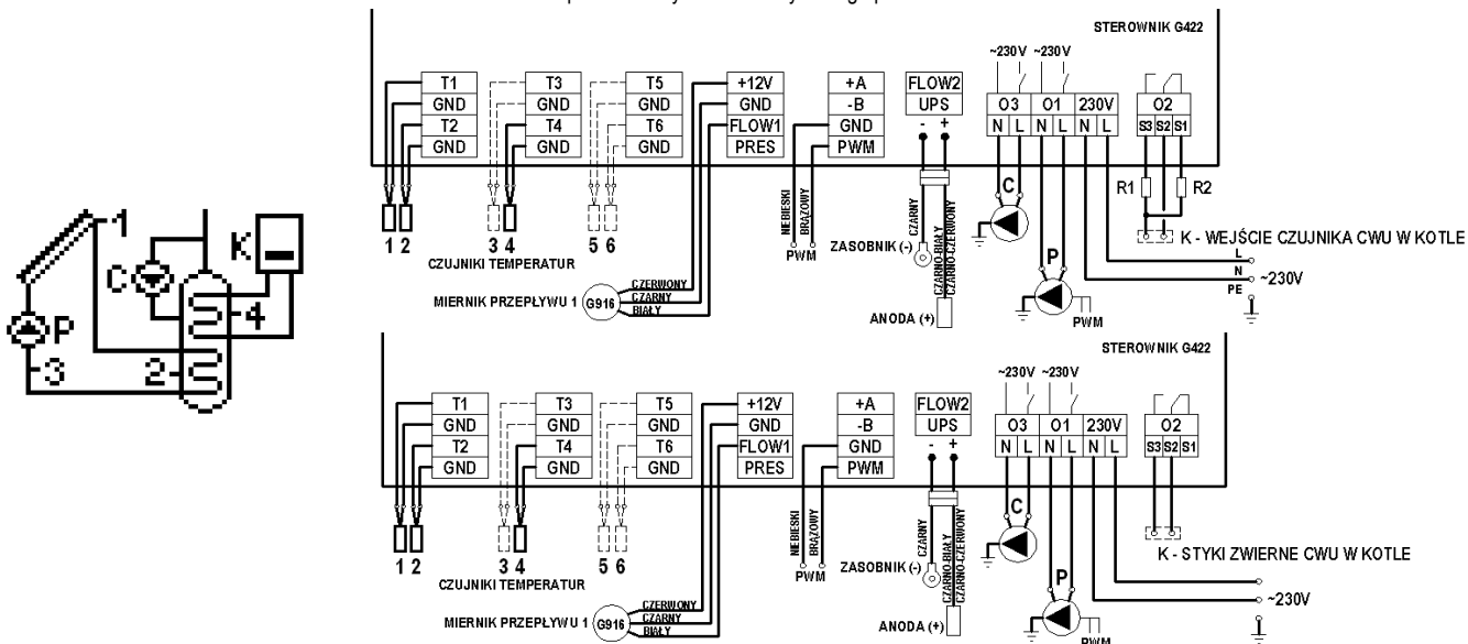
Schemat 3. Schemat ideowy oraz elektryczny instalacji nr 3.
