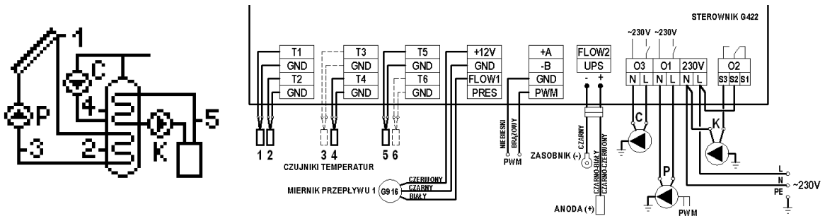
Schemat 6. Schemat ideowy oraz elektryczny instalacji nr 6.
