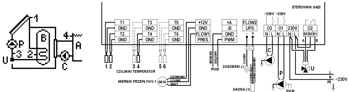
Schemat 9. Schemat ideowy oraz elektryczny instalacji układu nr 9.
