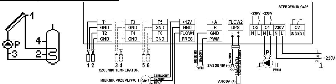
Schemat 1. Schemat ideowy oraz elektryczny instalacji nr 1.
