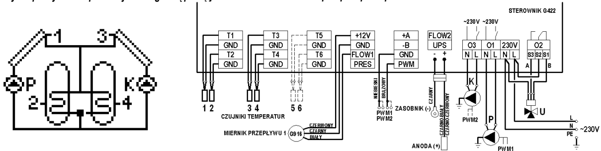
Schemat 16. Schemat ideowy oraz elektryczny instalacji układu nr 16.
