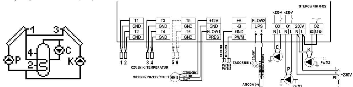
Schemat 15. Schemat ideowy oraz elektryczny instalacji układu nr 15.
