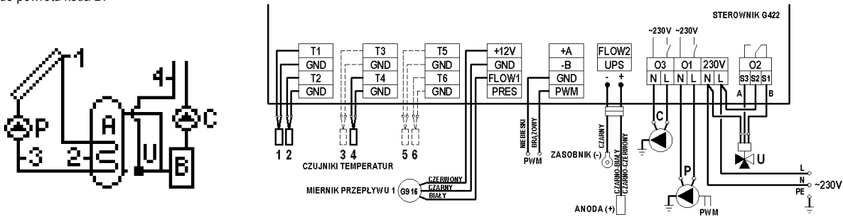
Schemat 13. Schemat ideowy oraz elektryczny instalacji układu nr 13.
