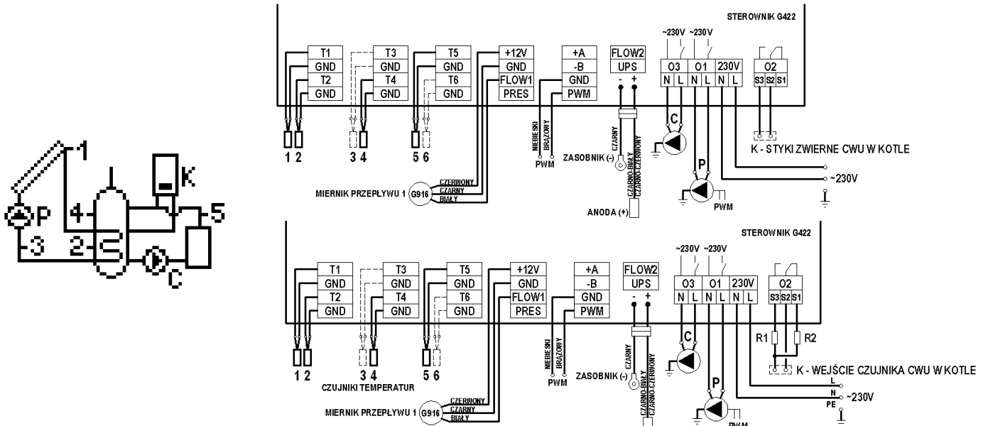
Schemat 14. Schemat ideowy oraz elektryczny instalacji układu nr 14.
