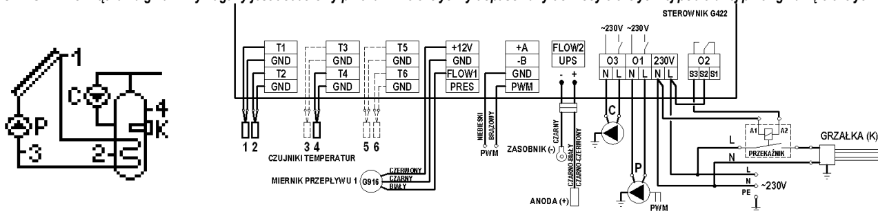
Schemat 4. Schemat ideowy oraz elektryczny instalacji nr 4.
