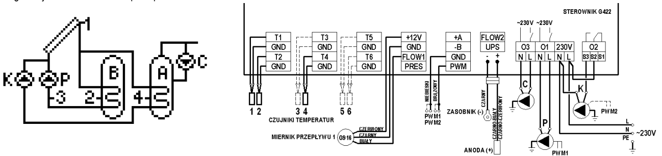
Schemat 12. Schemat ideowy oraz elektryczny instalacji układu nr 12.
