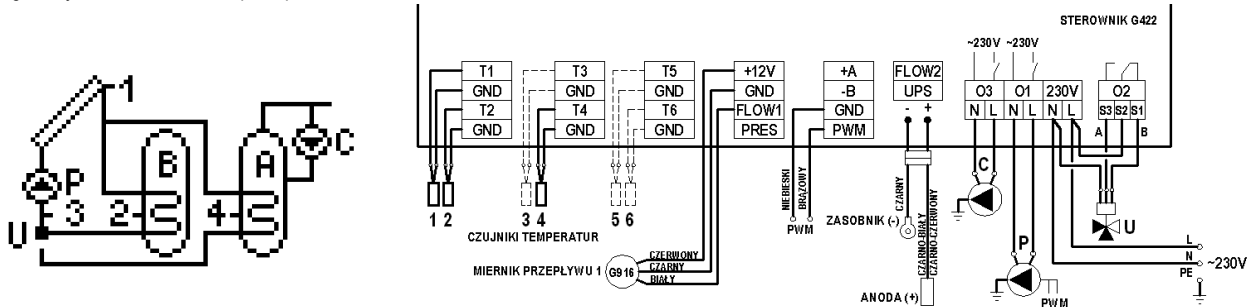
Schemat 11. Schemat ideowy oraz elektryczny instalacji układu nr 11.
