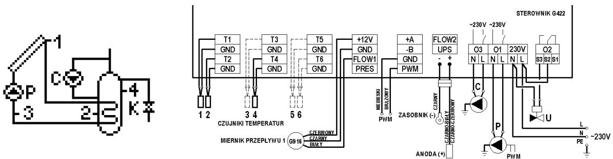
Schemat 17. Schemat ideowy oraz elektryczny instalacji układu nr 17.
