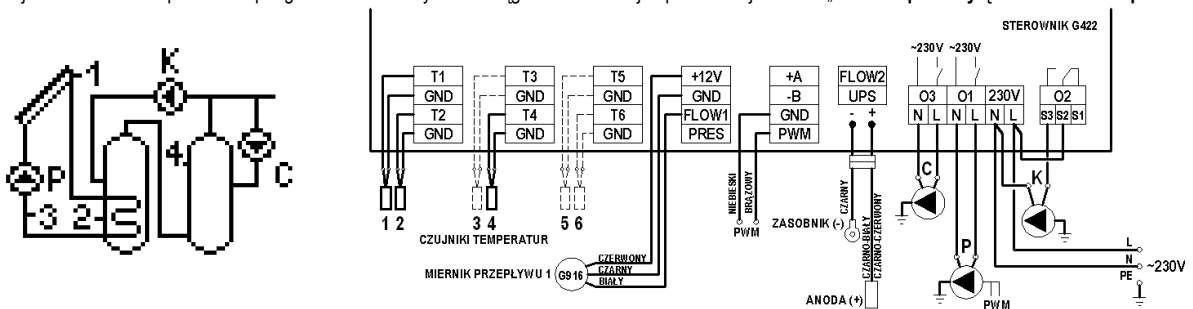
Schemat 7. Schemat ideowy oraz elektryczny instalacji nr 7.
