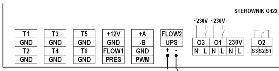
Rys. 1. Oznaczenia wejść i wyjść sterownika.
