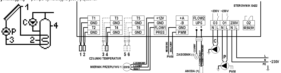
Schemat 2. Schemat ideowy oraz elektryczny instalacji nr 2.
