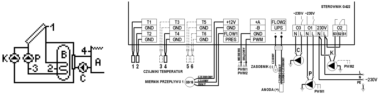
Schemat 10. Schemat ideowy oraz elektryczny instalacji nr 10.
