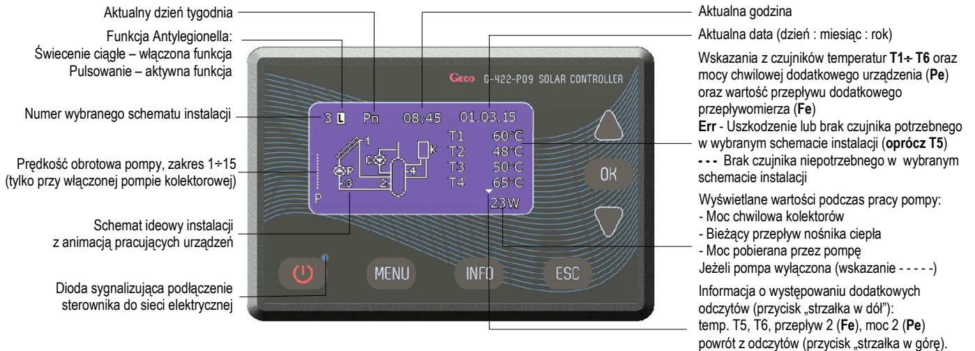
Rys. 2. Opis podstawowego ekranu na wyświetlaczu LCD
