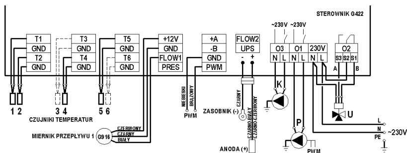
Schemat 19. Schemat ideowy oraz elektryczny instalacji układu nr 19.
