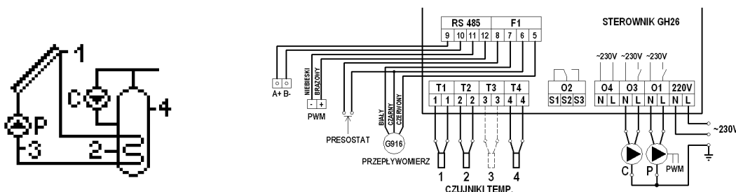
Schemat 2. Schemat ideowy oraz elektryczny instalacji nr 2.
