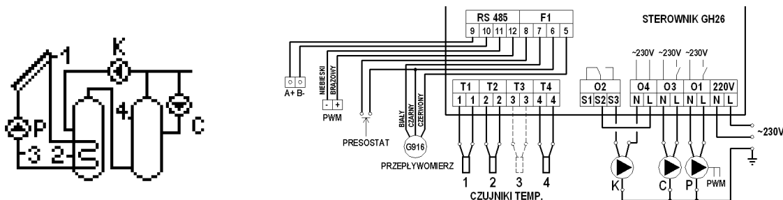
Schemat 7. Schemat ideowy oraz elektryczny instalacji nr 7.
