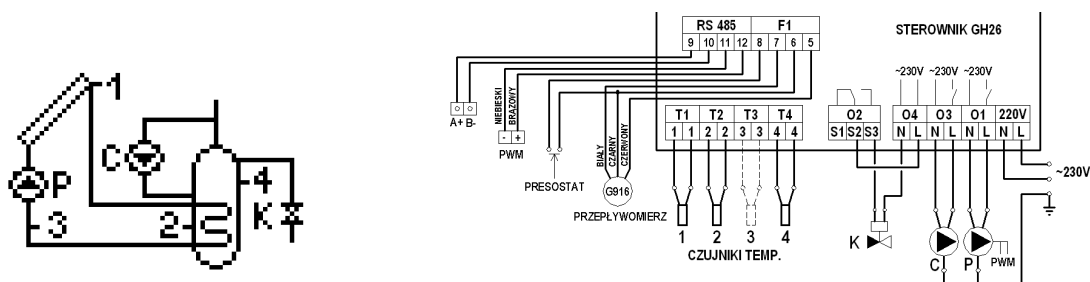
Rys. 19. Schemat ideowy oraz elektryczny instalacji układu nr 17.
