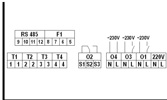
Rys. 1. Oznaczenie wejść i wyjść sterownika.
