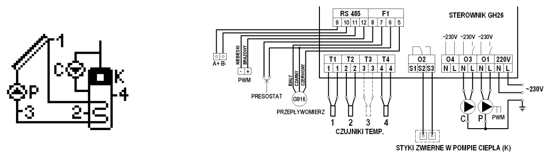
Schemat 5. Schemat ideowy oraz elektryczny instalacji nr 5.
