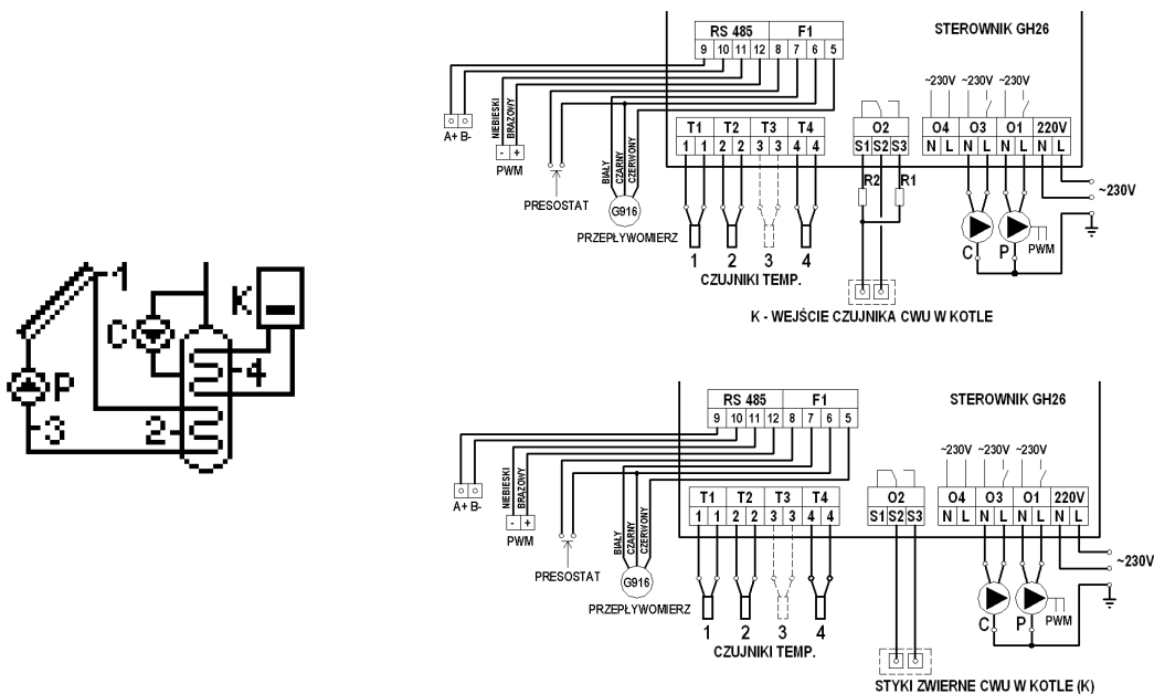
Schemat 3. Schemat ideowy oraz elektryczny instalacji nr 3.
