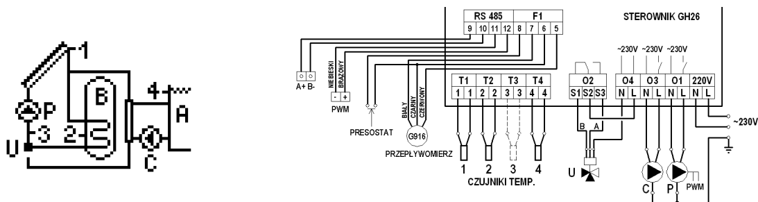
Schemat 9. Schemat ideowy oraz elektryczny instalacji nr 9.
