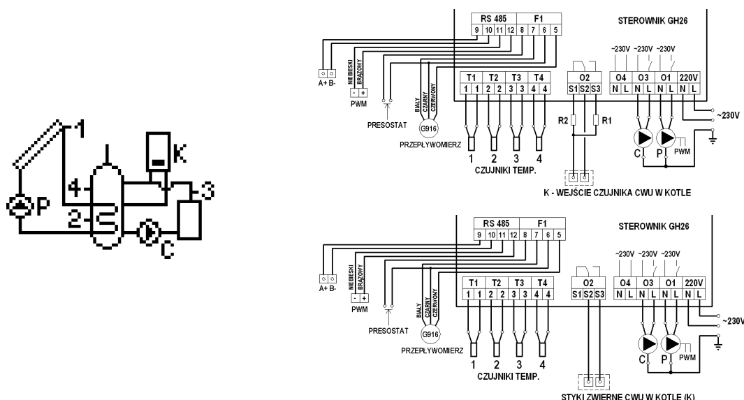
Schemat 14. Schemat ideowy oraz elektryczny instalacji układu nr 14.
