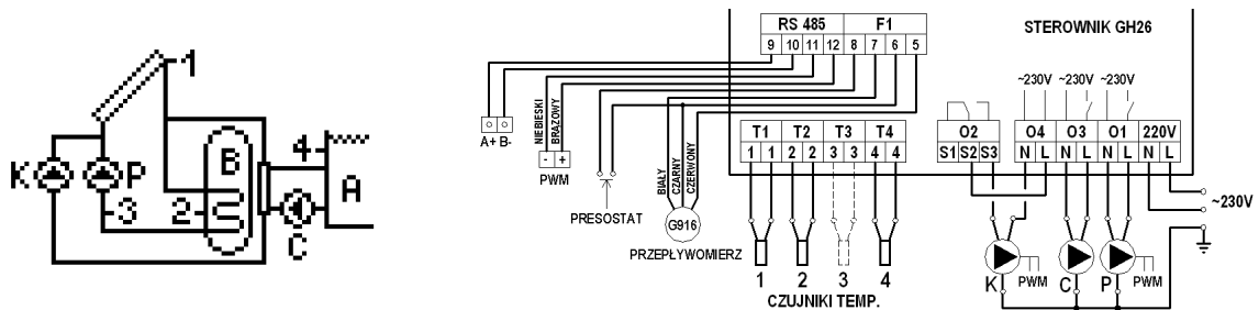
Schemat 10. Schemat ideowy oraz elektryczny instalacji nr 10.
