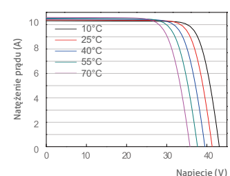
Krzywa prąd-napięcie JAM60S10-335/MR
