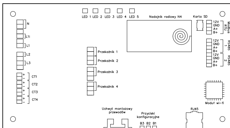
Rys. 3. Lokalizacja przycisków konfiguracyjnych B1 B2 B3, RJ45, ZASILANIE
