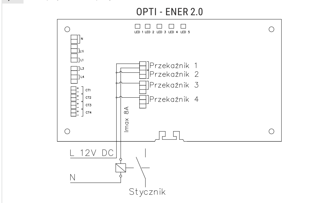
Rys. 9. Schemat podłączeń odbiorników pod styki zwierne.
