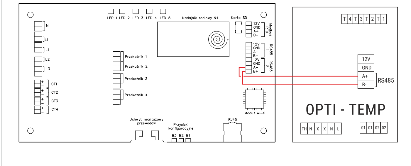
Rys. 7. Schemat podłączenia urządzenia OPTI-TEMP
