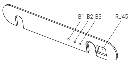
Rys. 3. Lokalizacja przycisków konfiguracyjnych B1 B2 B3, RJ45, ZASILANIE
