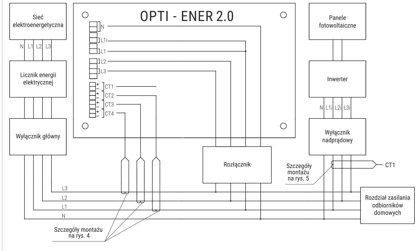
Rys. 6. Sposób montażu układu pomiarowego
