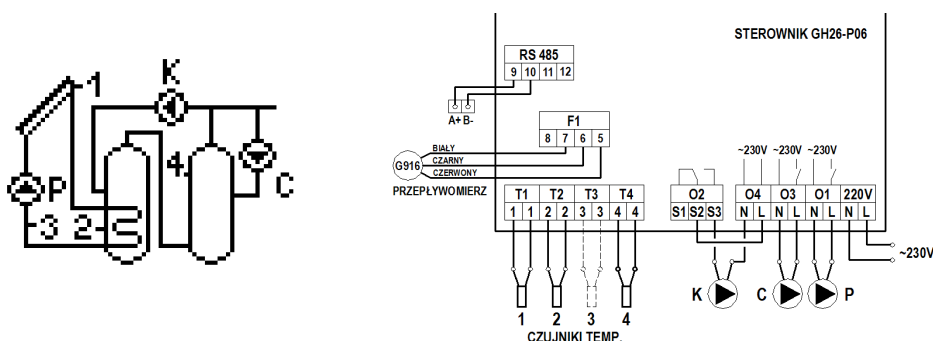
Rys. 9. Schemat ideowy oraz elektryczny instalacji nr 7.
