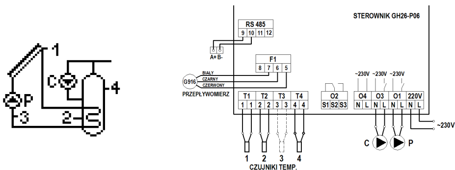
Rys. 4. Schemat ideowy oraz elektryczny instalacji nr 2.
