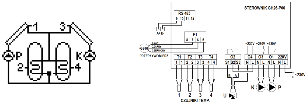
Rys. 18. Schemat ideowy oraz elektryczny instalacji układu nr 16.
