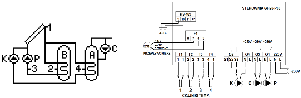
Rys. 14. Schemat ideowy oraz elektryczny instalacji układu nr 12.
