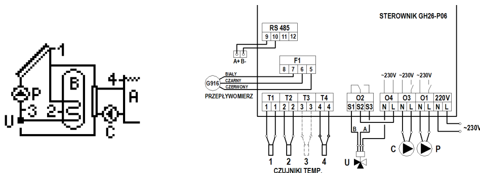
Rys. 11. Schemat ideowy oraz elektryczny instalacji nr 9.
