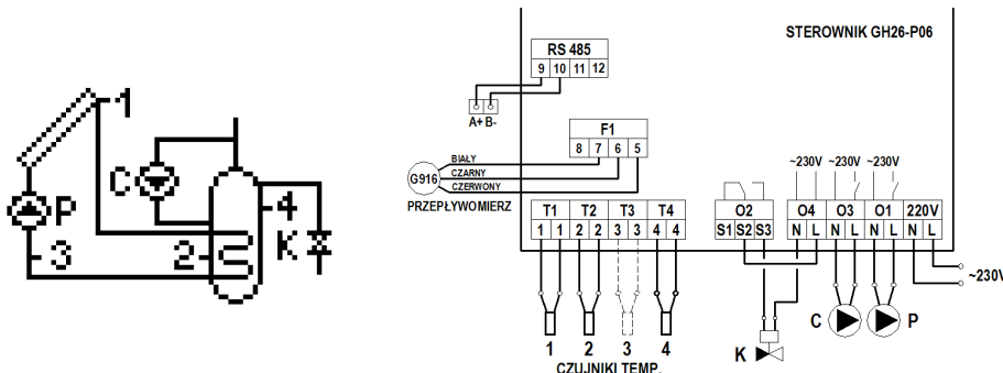
Rys. 19. Schemat ideowy oraz elektryczny instalacji układu nr 17.
