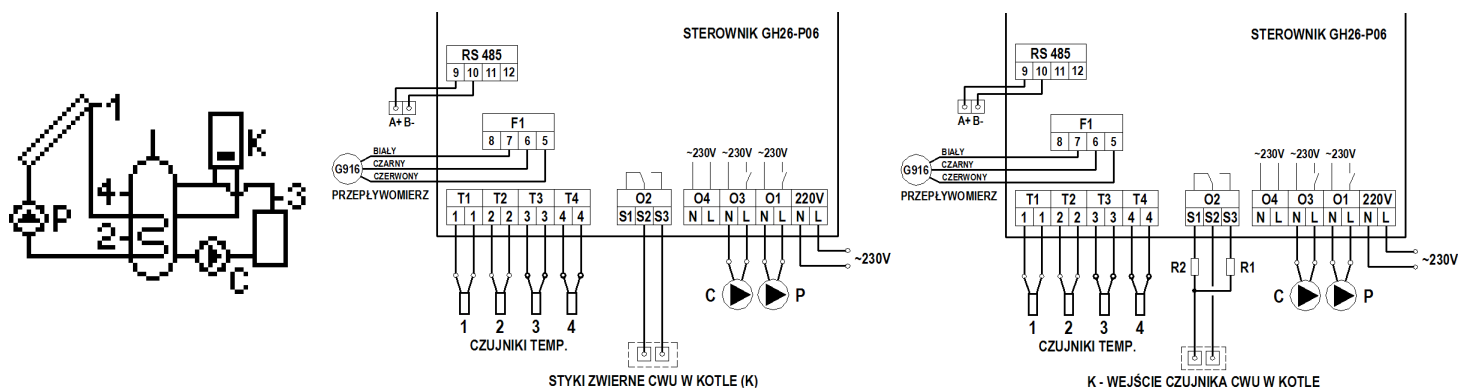
Rys. 16. Schemat ideowy oraz elektryczny instalacji układu nr 14.
