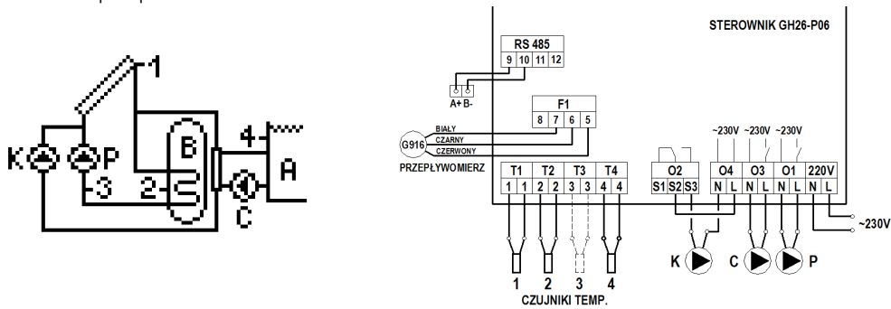
Rys. 12. Schemat ideowy oraz elektryczny instalacji nr 10.
