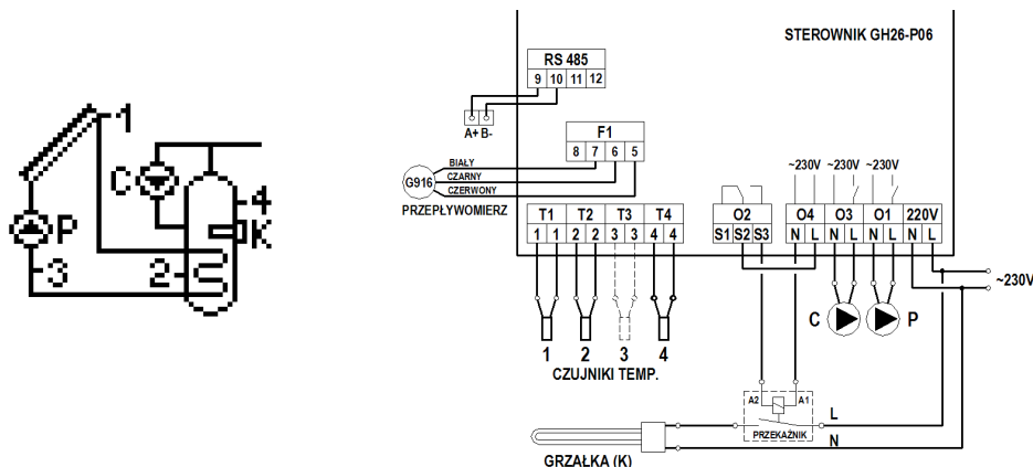
Rys. 6. Schemat ideowy oraz elektryczny instalacji nr 4.
