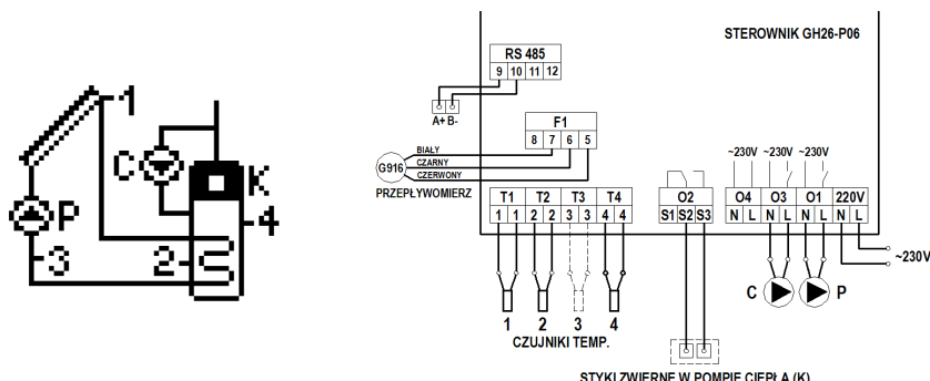
Rys. 7. Schemat ideowy oraz elektryczny instalacji nr 5.
