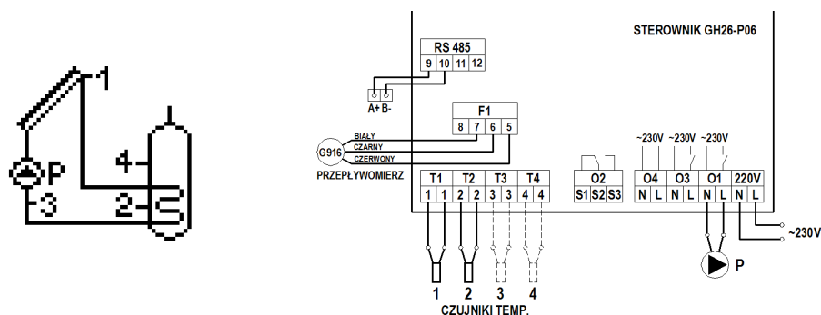
Rys. 3. Schemat ideowy oraz elektryczny instalacji nr 1.
