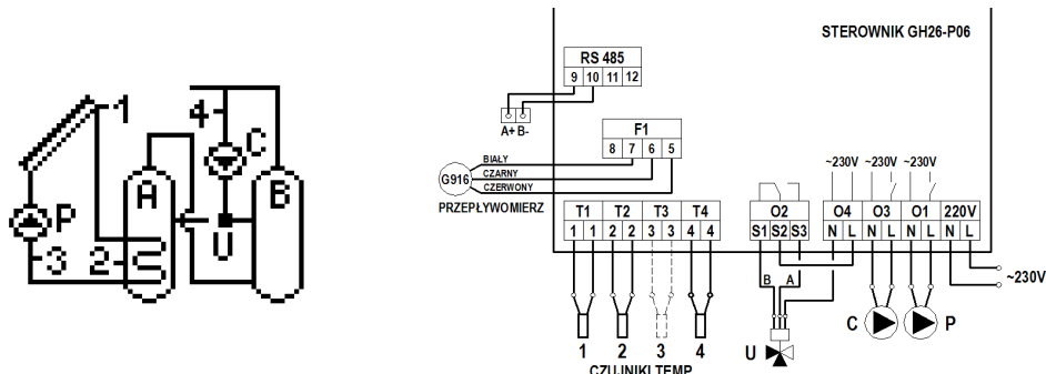
Rys. 10. Schemat ideowy oraz elektryczny instalacji układu nr 8.
