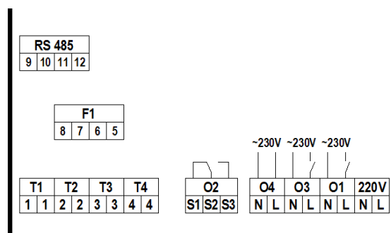
Rys. 1. Oznaczenie wejść i wyjść sterownika.
