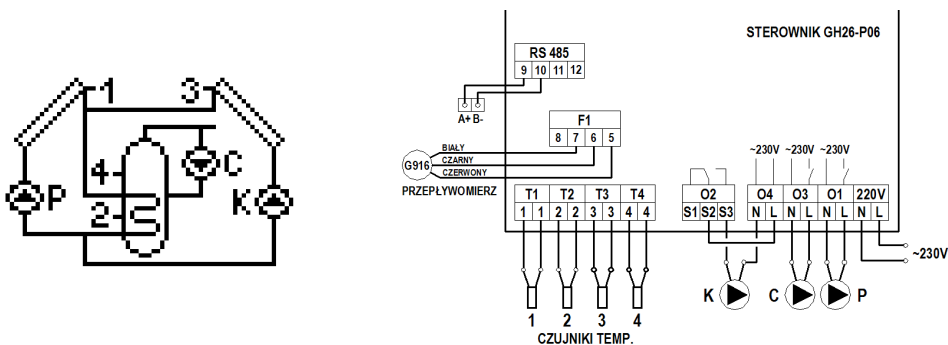
Rys. 17. Schemat ideowy oraz elektryczny instalacji układu nr 15.
