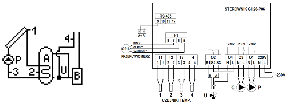
Rys. 15. Schemat ideowy oraz elektryczny instalacji układu nr 13.
