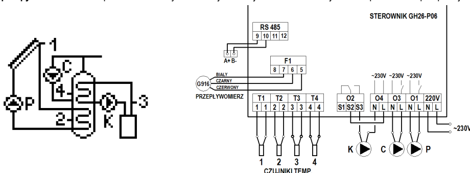
Rys. 8. Schemat ideowy oraz elektryczny instalacji nr 6.
