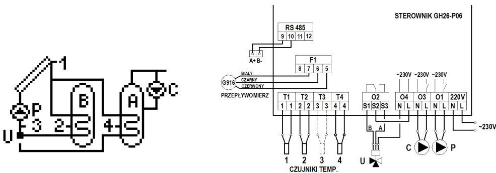
Rys. 13. Schemat ideowy oraz elektryczny instalacji układu nr 11.
