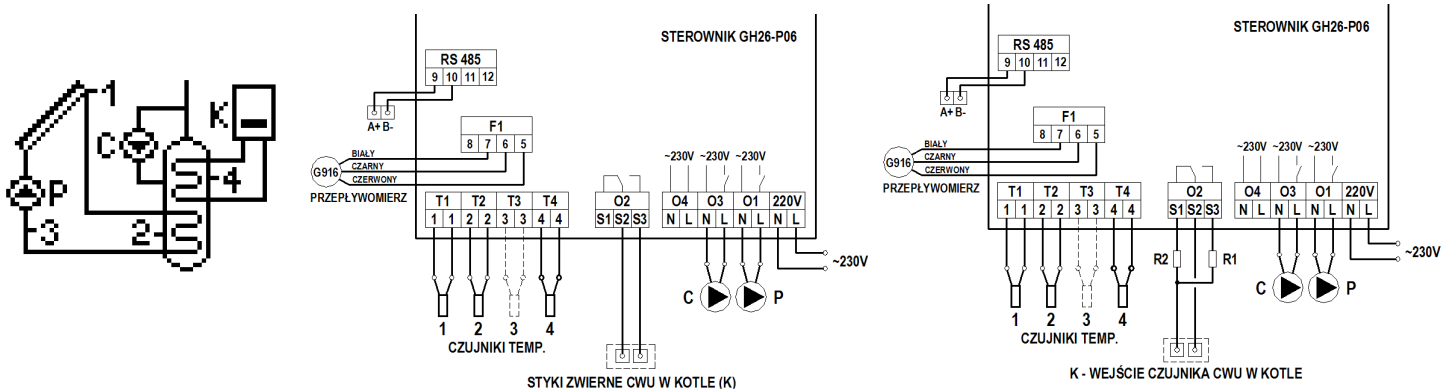
Rys. 5. Schemat ideowy oraz elektryczny instalacji nr 3.
