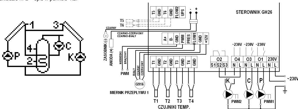
Schemat 15. Schemat ideowy oraz elektryczny instalacji układu nr 15.
