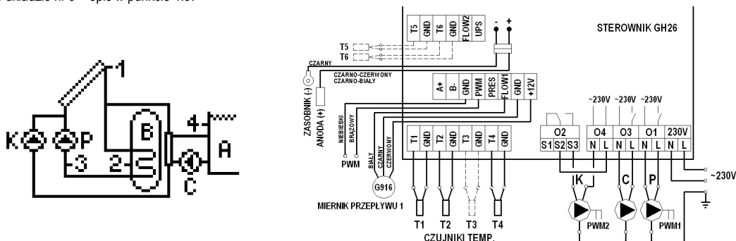
Schemat 10. Schemat ideowy oraz elektryczny instalacji nr 10.
