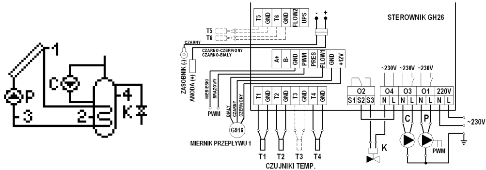
Schemat 17. Schemat ideowy oraz elektryczny instalacji układu nr 17.
