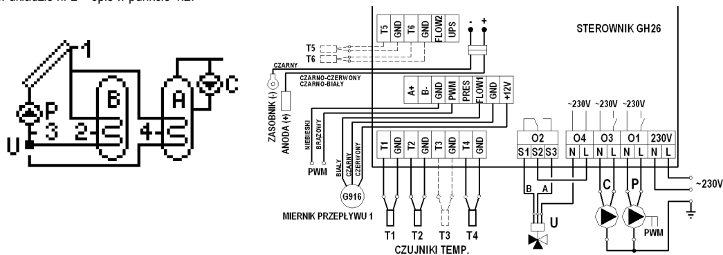
Schemat 11. Schemat ideowy oraz elektryczny instalacji układu nr 11.
