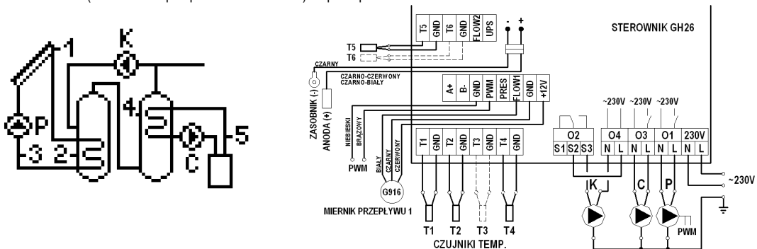
Schemat 18. Schemat ideowy oraz elektryczny instalacji układu nr 18.
