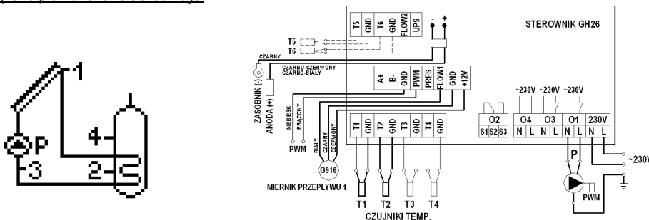
Schemat 1. Schemat ideowy oraz elektryczny instalacji nr 1.
