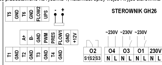
Rys. 1. Oznaczenia wejść i wyjść sterownika.
