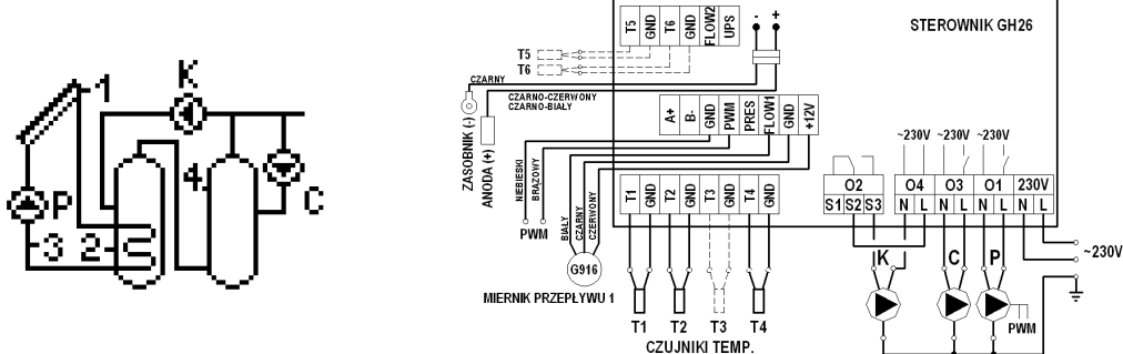
Schemat 7. Schemat ideowy oraz elektryczny instalacji nr 7.
