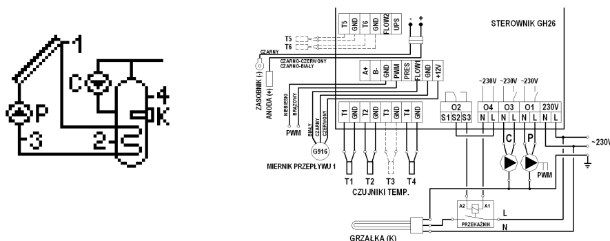
Schemat 4. Schemat ideowy oraz elektryczny instalacji nr 4.
