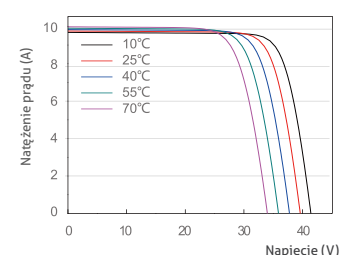
Krzywa prąd-napięcie JAM60S01-310/PR
