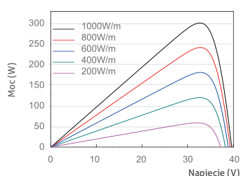
Krzywa moc-napięcie JAM60S01-310/PR
