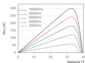
Krzywa moc-napięcie JAM60S01-315/PR
