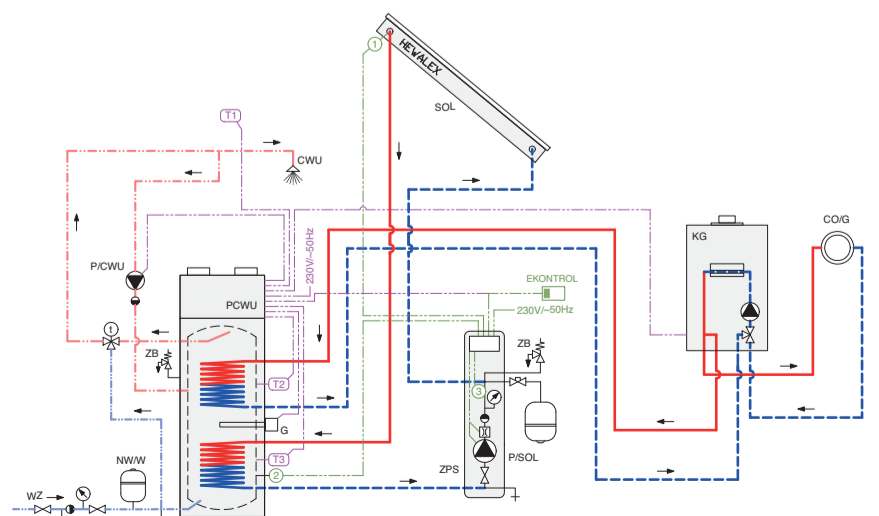
Fot. 4. Schemat systemu grzewczego z gazowym kotłem wiszącym (KG), pompą ciepła wody użytkowej (PCWU) oraz instalacją solarną. Zarządzanie podgrzewaniem wody użytkowej realizowane jest przez sterownik pompy ciepła (Hewalex G-426).
