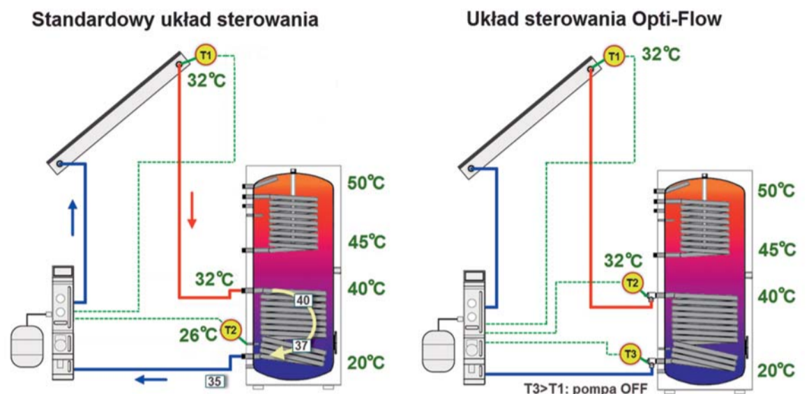
Fot. 2. Porównanie zasady pracy instalacji solarnej: standardowej oraz w funkcji Opti-Flow. Możliwe w standardowej instalacji niepożądane zjawisko „wyrzucania” ciepła jest wyeliminowane w funkcji Opti-Flow.
