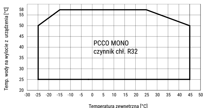
Pole pracy sprężarki dla pompy ciepła z czynnikiem R32.
