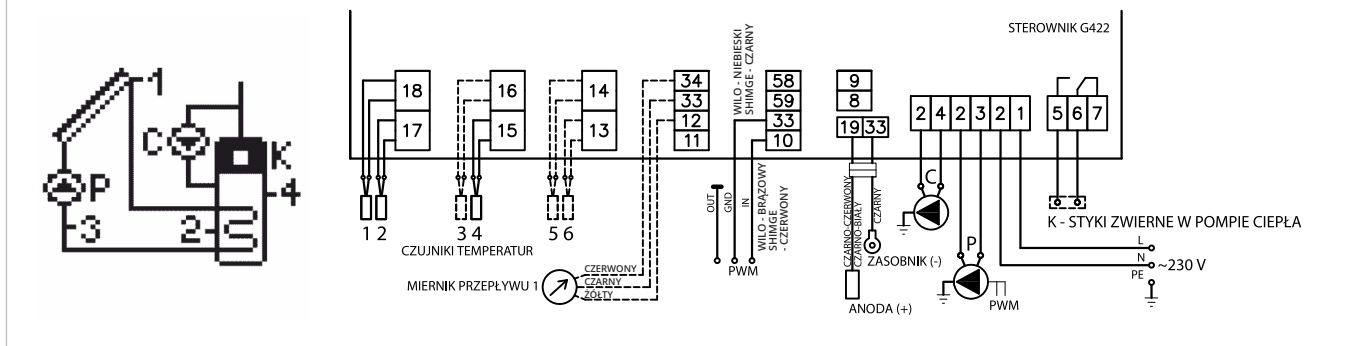
Schemat 5. Schemat ideowy oraz elektryczny instalacji nr 5.
