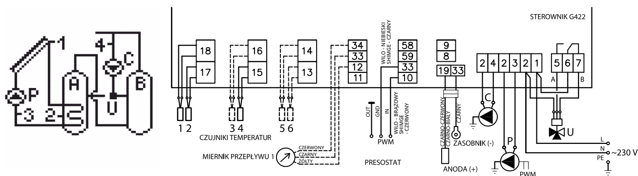
Schemat 8. Schemat ideowy oraz elektryczny instalacji nr 8.
