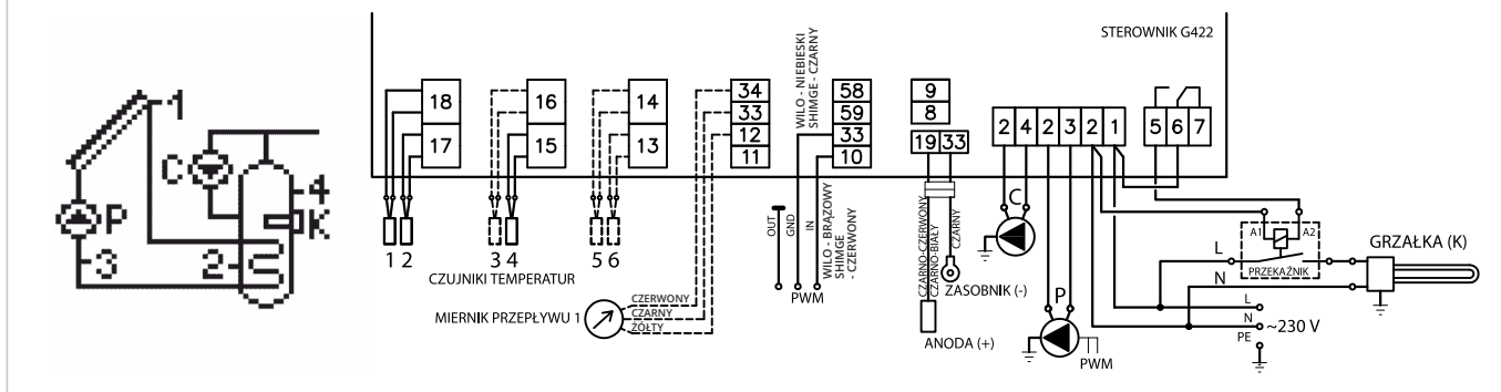
Schemat 4. Schemat ideowy oraz elektryczny instalacji nr 4.
