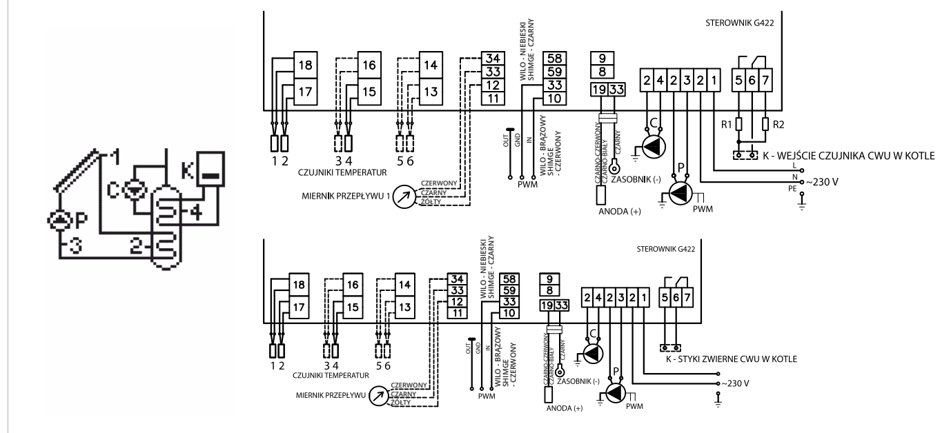
Schemat 3. Schemat ideowy oraz elektryczny instalacji nr 3.
