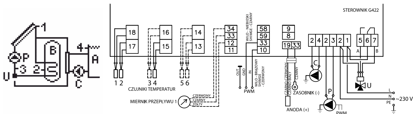
Schemat 9. Schemat ideowy oraz elektryczny instalacji nr 9.
