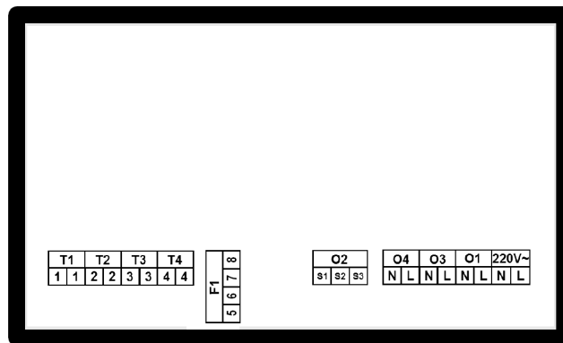
Rys. 1. Oznaczenie wejść i wyjść sterownika.
