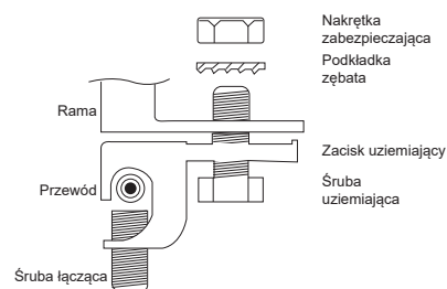
Rys. 6: Metody montażu
