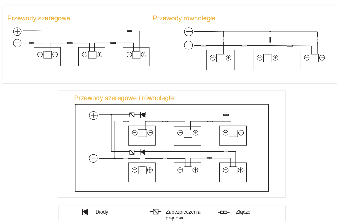
Rys. 4: Schematy elektryczne połączeń szeregowych i równoległych
