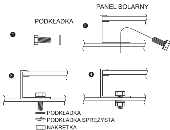
Rysunek 2 Szczegóły dotyczące mocowań
