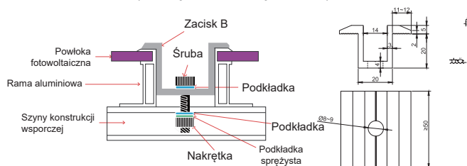
Zacisk B Zacisk używany na module środkowym
