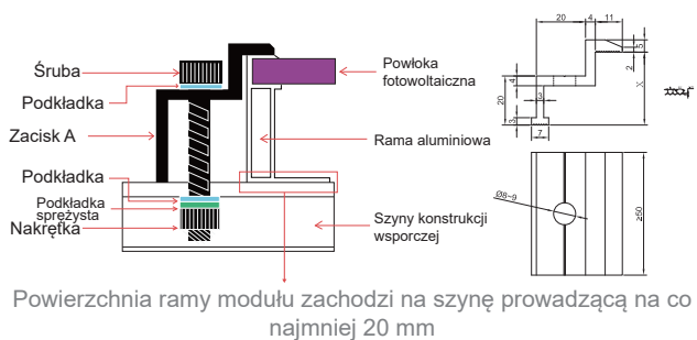
Zacisk A Zacisk używany na module bocznym (X = wysokość ramy modułu)
