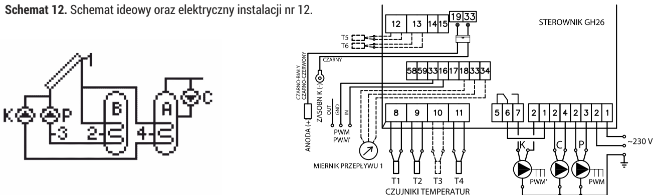
Schemat 12. Schemat ideowy oraz elektryczny instalacji nr 12.
