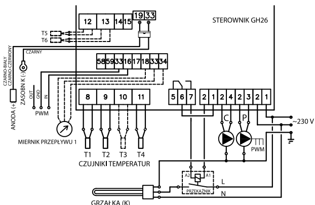
Schemat 4. Schemat ideowy oraz elektryczny instalacji nr 4.
