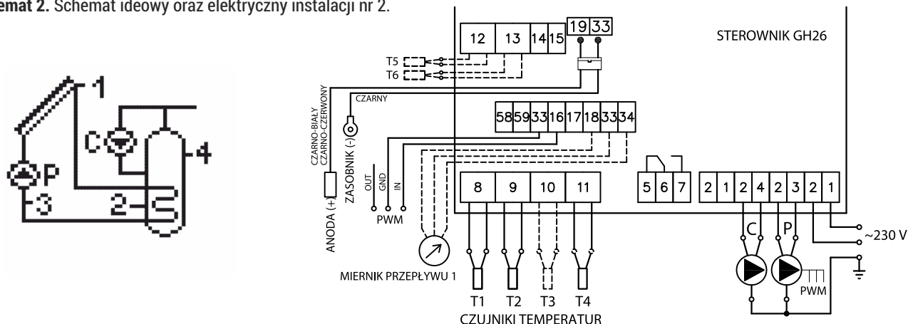
Schemat 2. Schemat ideowy oraz elektryczny instalacji nr 2.
