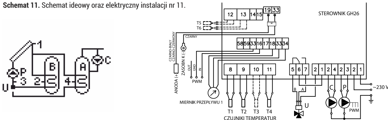
Schemat 11. Schemat ideowy oraz elektryczny instalacji nr 11.
