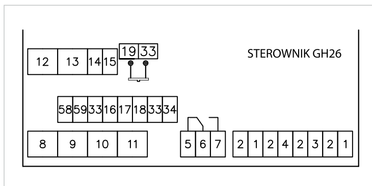
Rys. 1. Oznaczenia wejść i wyjść sterownika.
