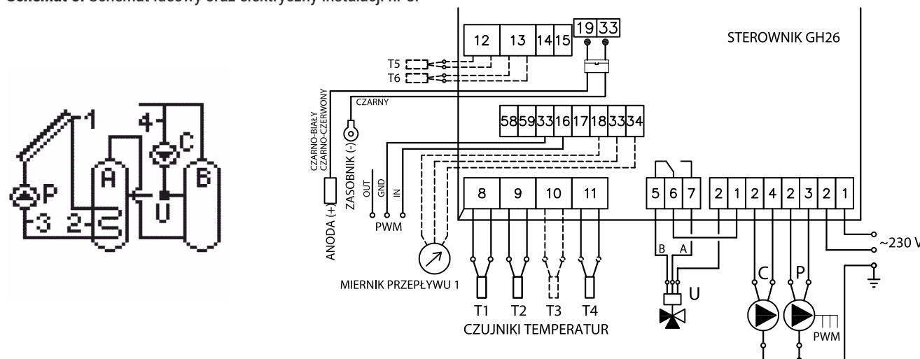
Schemat 8. Schemat ideowy oraz elektryczny instalacji nr 8.
