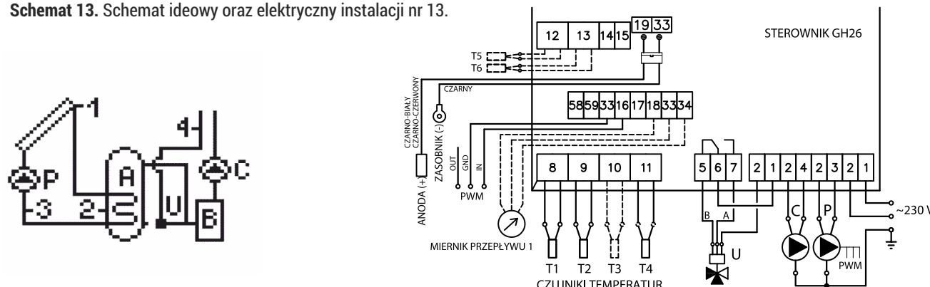
Schemat 13. Schemat ideowy oraz elektryczny instalacji nr 13.
