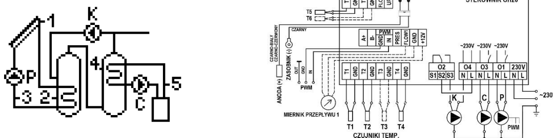
Schemat 18. Schemat ideowy oraz elektryczny instalacji układu nr 18.
