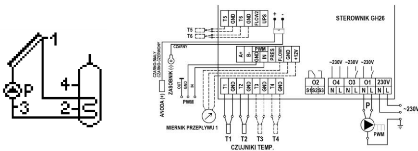
Schemat 1. Schemat ideowy oraz elektryczny instalacji nr 1.
