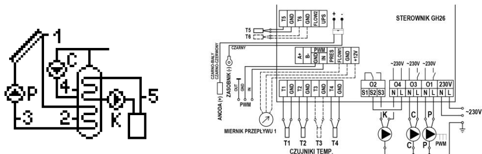
Schemat 6. Schemat ideowy oraz elektryczny instalacji nr 6.
