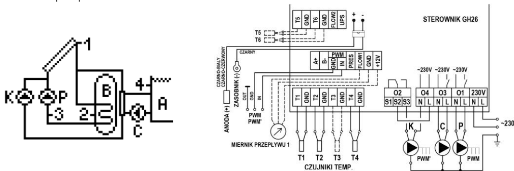
Schemat 10. Schemat ideowy oraz elektryczny instalacji nr 10.
