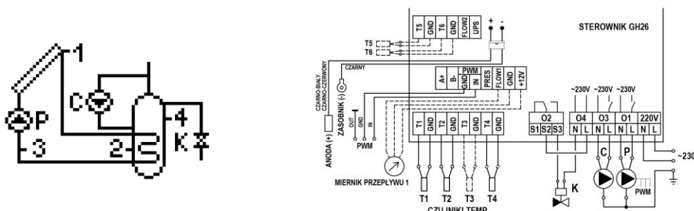
Schemat 17. Schemat ideowy oraz elektryczny instalacji układu nr 17.
