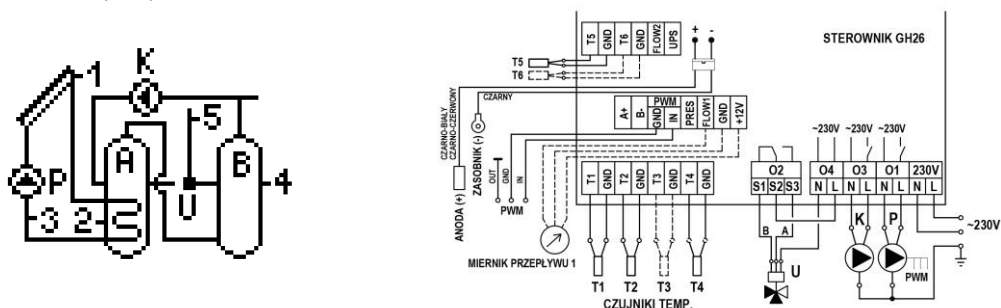
Schemat 19. Schemat ideowy oraz elektryczny instalacji układu nr 19.
