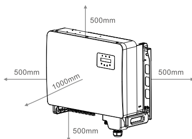
Rysunek 5.2 Odstęp montażowy falownika
