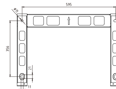
Rysunek 5.3 Montaż naścienny falownika
