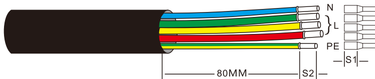
Rysunek 5.18 Zdjęcie izolacji z kabla prądu zmiennego
