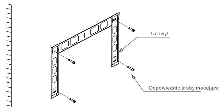
Rysunek 5.4 Montaż naścienny falownika
