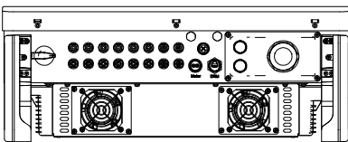
Rysunek 5.17 Podłączenie złącza DC do falownika
