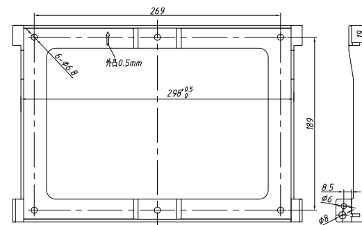
Rysunek 5.3 Montaż naścienny falownika
