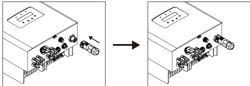
Rysunek 5.24 Podłącz złącze AC do falownika
