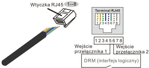
Rysunek 5.31 Zdejmij warstwę izolacyjną i podłącz do wtyczki RJ45
