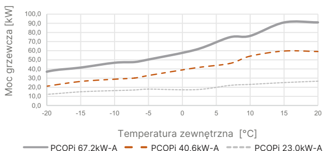
Moc grzewcza przy temp. wody 55°C dla maksymalnej częstotliwości sprężarki
