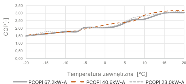
COP przy temp. wody 55°C dla maksymalnej częstotliwości sprężarki
